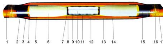
1 铜屏蔽带 2 外半导体层 3、密封胶 4、应力疏散胶 5、应力控制管 6、XLPE绝缘 7 内半导体层 8、导体 9、半导电带 10、连接管 11 填充胶 12 内绝缘管 13、外绝缘管 14、半导管 15、铜编织线 16、扎线 17 铜屏蔽网
