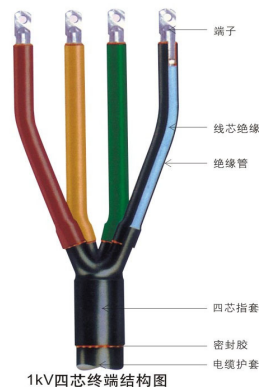
1kV四芯终端结构图
